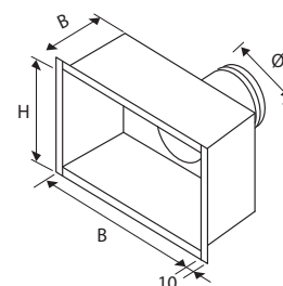
Povezovalna komora KK-H
