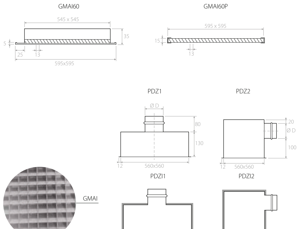
Povezovalna komora z izolacijo 6 mm.
